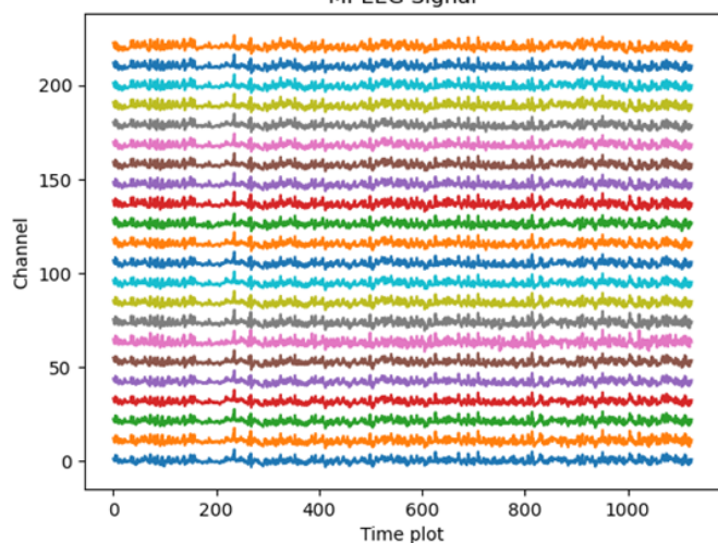
MI-EEG Signal
