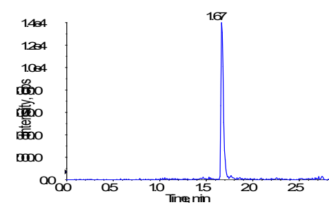
Bupropion-LLOQ
