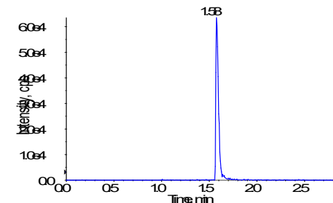
O-desmethylvenlafaxine-LLOQ
