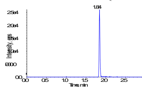
Doxepin-LLOQ
