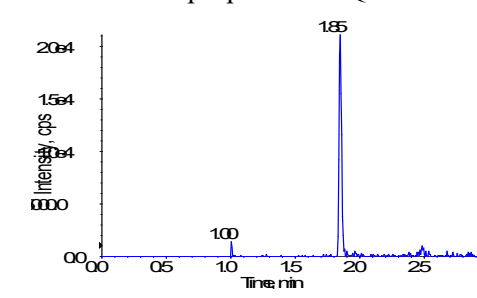
Mianserin-LLOQ
