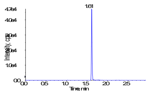
Mirtazapine-LLOQ
