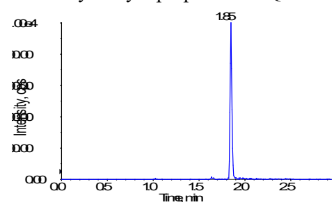
Nordoxepin-LLOQ
