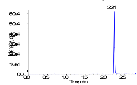
Agomelatine-LLOQ
