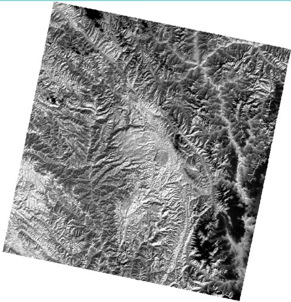
Fig.6. LST results
