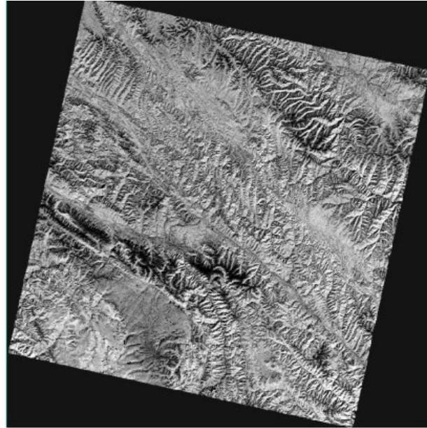
Fig.3. NDVI
